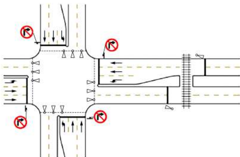
Рисунок К.3 - Схема взаимного расположения железнодорожного переезда и пересечения дорог Расчет длины очереди перед железнодорожным переездом проводится по формуле
